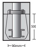
inground base (23)
